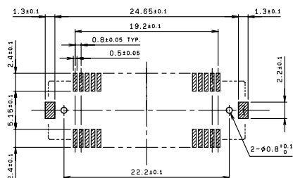
基板取り付け寸法 MOUNTING LAYOUT
