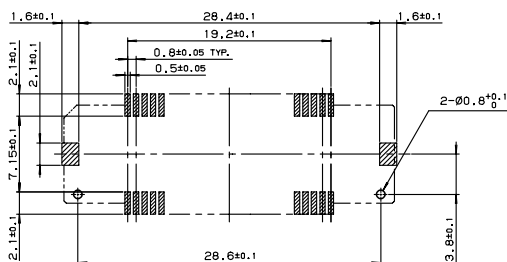
基板取り付け寸法 MOUNTING LAYOUT
