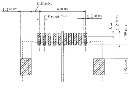
基板取り付け寸法 MOUNTING LAYOUT
