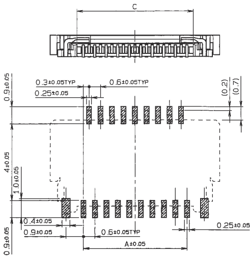
推奨基板パターン (MOUNTING LAYOUT)
