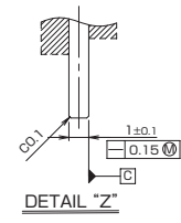
推奨メモリー基板寸法 RECOMMENDED MEMORY BOARD LAYOUT
