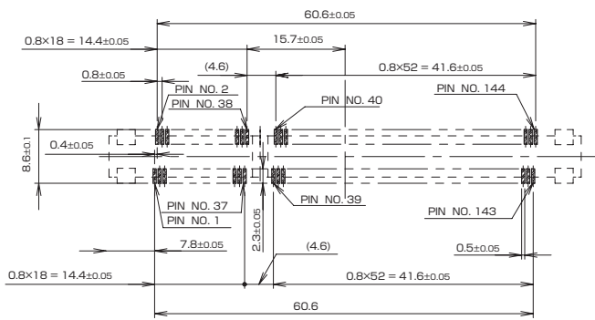
基板取付寸法 MOUNTING LAYOUT
