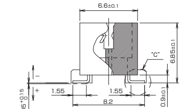
SECT. B-B (インシュレータ底面からコンタクトの突出) (PROJECTION OF THE BOTTOM OF INSULATOR CONTACT FROM THE BOTTOM OF INSULATOR)
