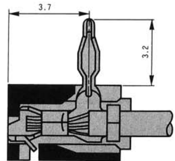
水平型装着断面 Right Angle Type Cross Cut Section
